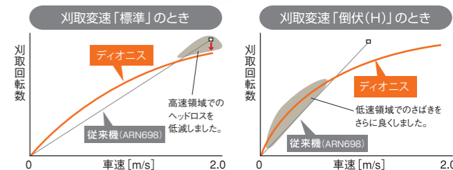
■刈取回転数と車速
