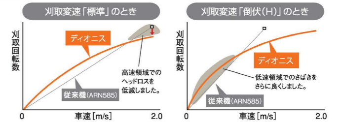
■刈取回転数と車速
