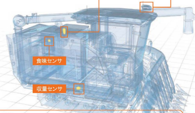
こく粒流量センサ
